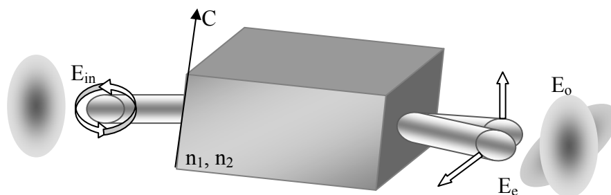
Рис. 1. Схема распространения сингулярного пучка с эллиптическим сечением в анизотропной среде с показателями преломления n_1, n_2 . E_{in} – падающий циркулярно поляризованный свет, E_e, E_o , – необыкновенный и обыкновенный пучки соответственно.
