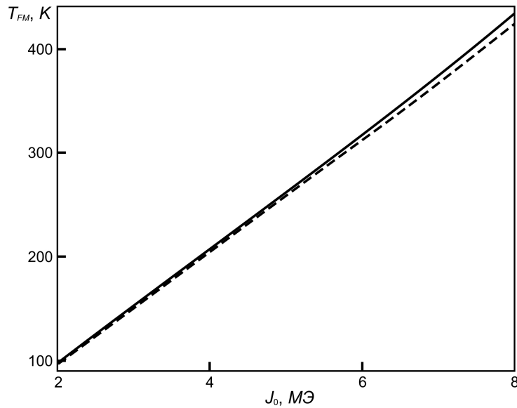
Рис. 1. Зависимость температуры фазового перехода T_{FM} от величины константы гейзенберговского обменного взаимодействия J_0 при различных значениях параметра магнитоупругой связи b_0 . Сплошная линия соответствует b_0 = 1500 Э, пунктирная – 150 Э.
