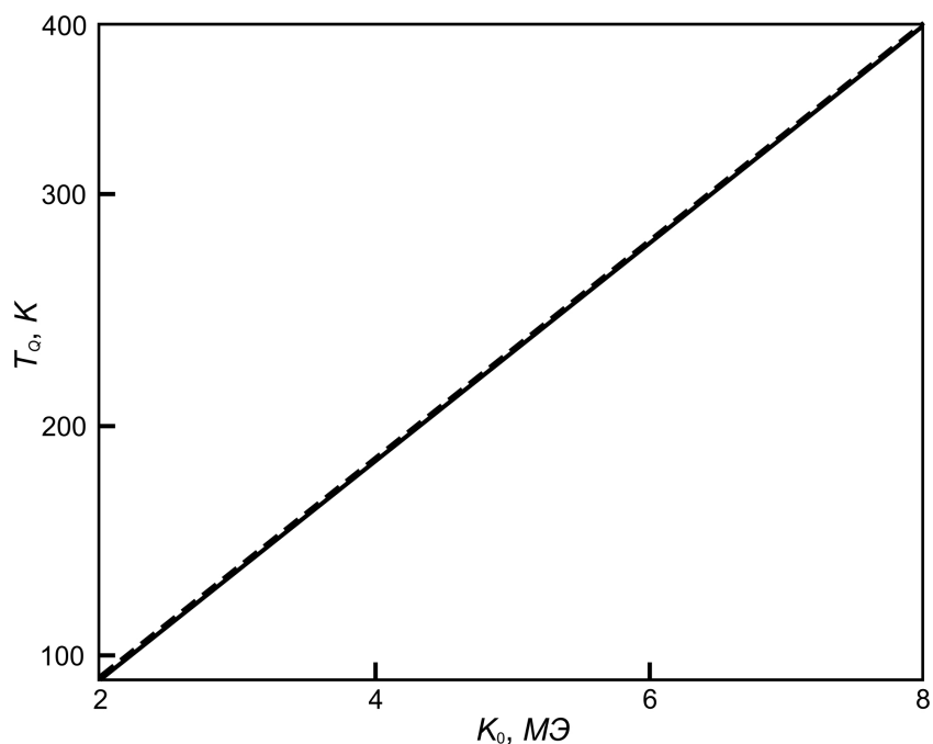
Рис. 2. Зависимость температуры фазового перехода T_Q от величины константы биквадратичного обменного взаимодействия K_0 при различных значениях параметра магнитоупругой связи b_0 . Сплошная линия соответствует b_0 = 1500 Э, пунктирная – 150 Э.
